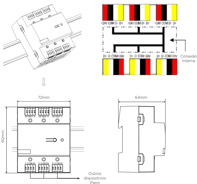
Figura 2. Dimensões e Ligação Elétrica
