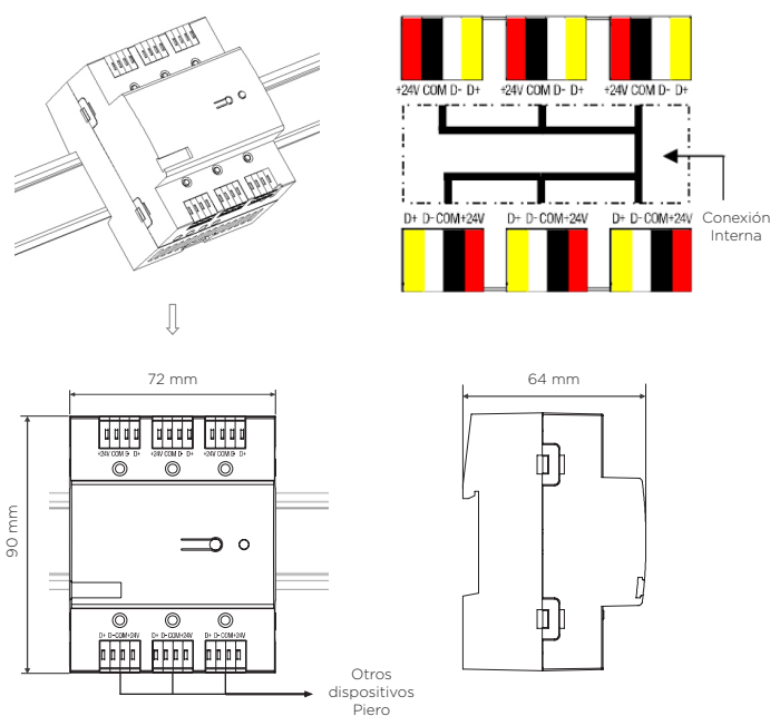
Figura 2. Dimensiones y Conexión Eléctrica
